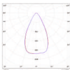
K60 - угол раскрытия 60°
